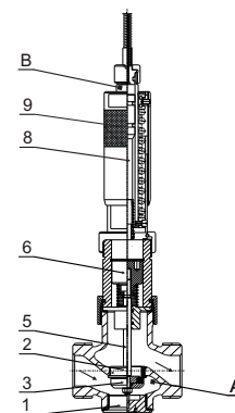
Zwór otwierający
