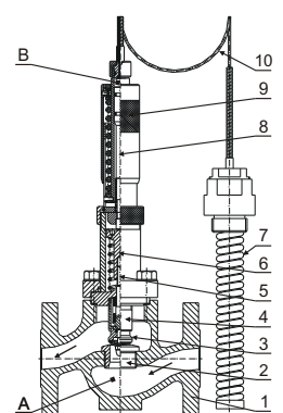
Zwór zamykający
