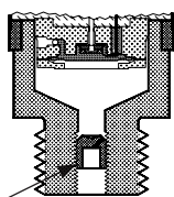
Tłumik pulsacji
