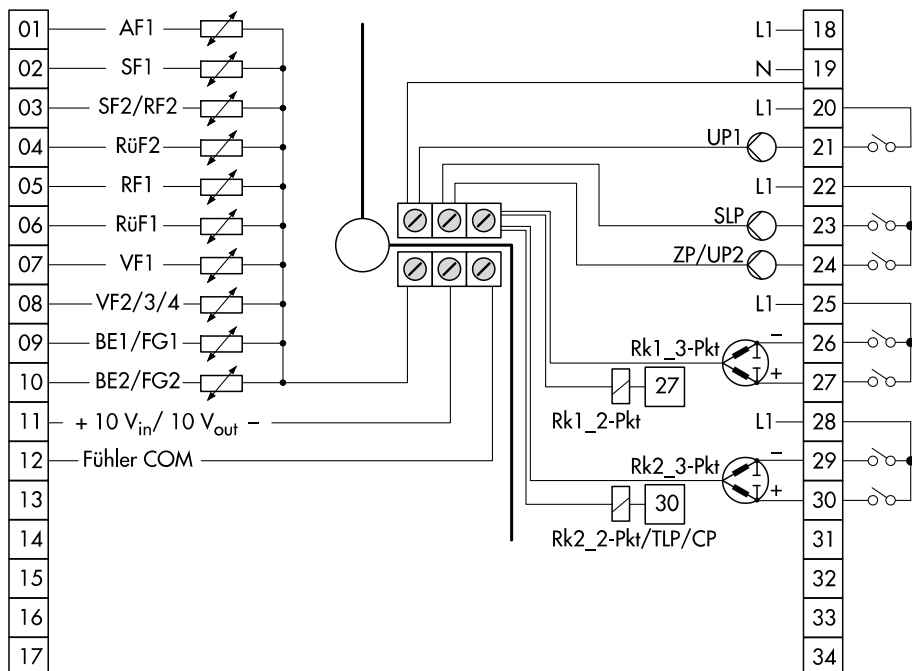
Rys. 3 · Przyporządkowanie zacisków regulatora TROVIS 5573 ze standardową podstawką
