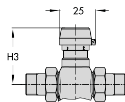
wykonanie z kapturkiem ze skalą do nastawy wartości zadanej przepływu
